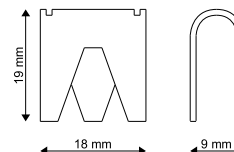
Klips zaciskowy
